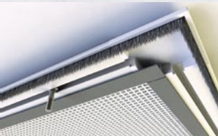
Bürstendichtung nach unten für eine saubere Abdichtung zum Lichtschacht und klapperfreies Begehen
