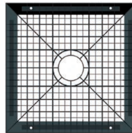
Seitenteil mit ausgesägter Öffnung DN 110
