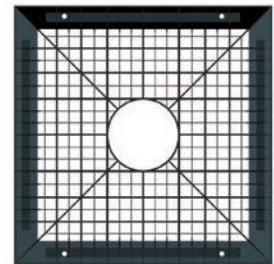
Seitenteil mit ausgesägter Öffnung DN 150
